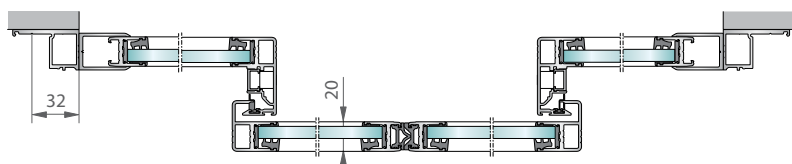
Montaggio su architrave
