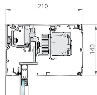
a 1 e 2 ante: Impianti senza anta fissa con profilo di montaggio
