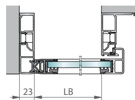
Montaggio a parete
