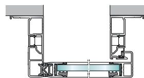
Montaggio su architrave
