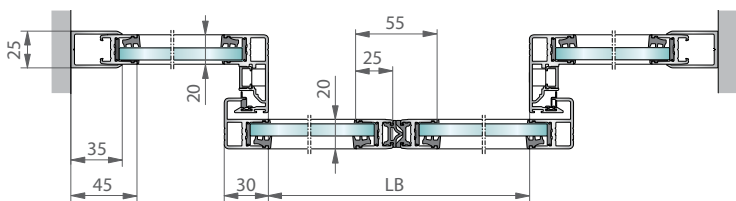
Montaggio su architrave
