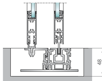
Guida a pavimento incassata
