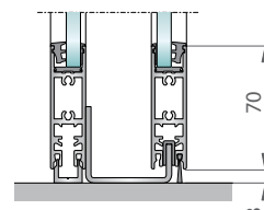
Guida a pavimento esterna
