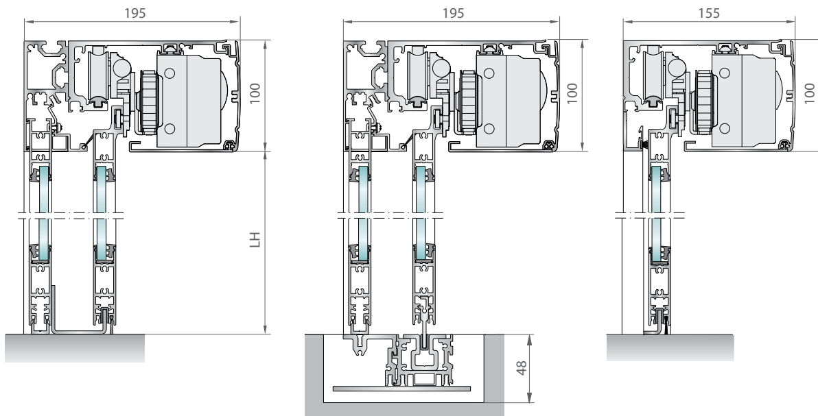
a 1 e 2 ante: Impianti con anta fissa e guida a pavimento esterna
